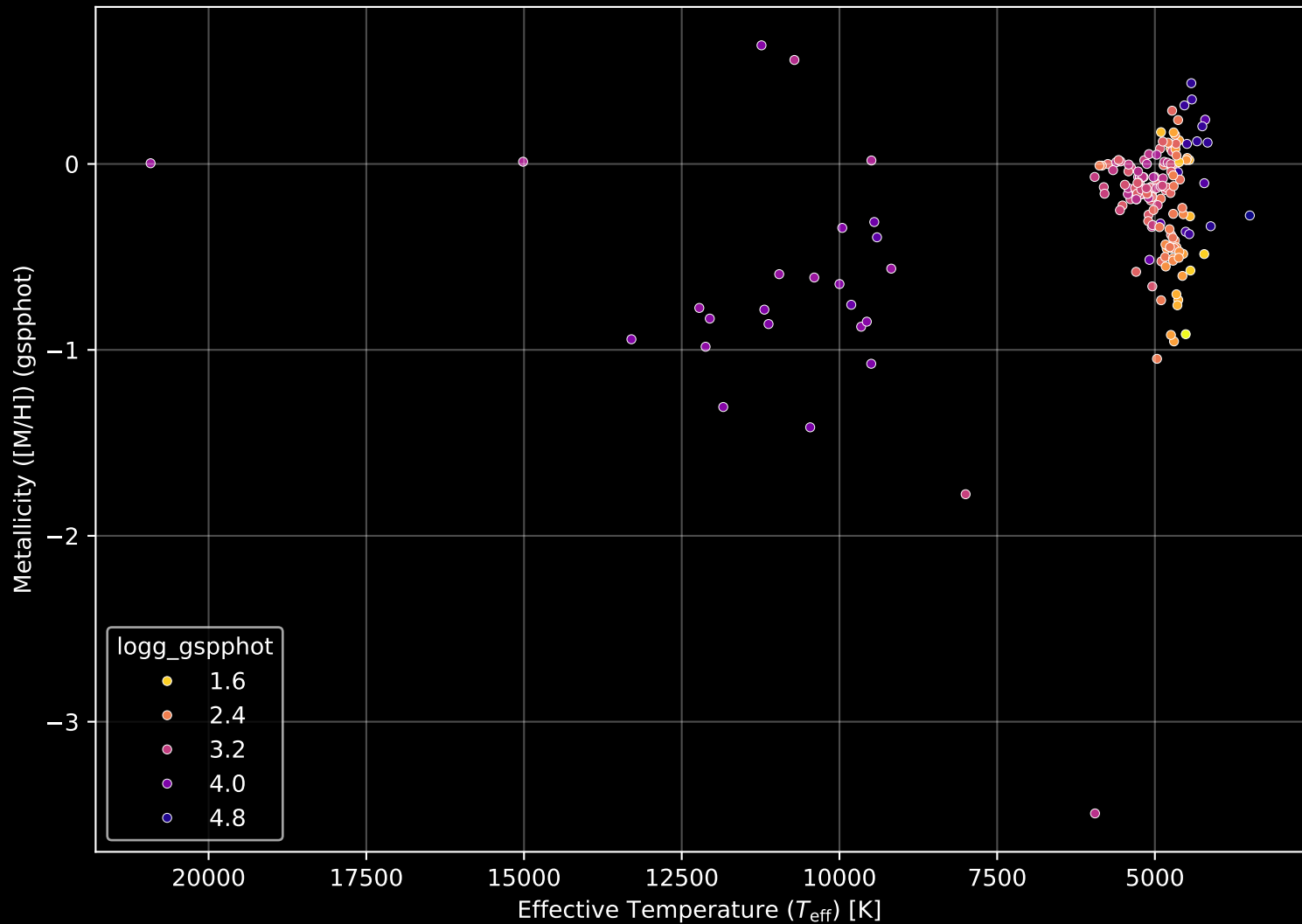
APOGEE DR17 Field: [214+04] Stellar Population Parameters (n= 179)
